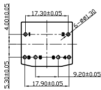
PCB板安装图
